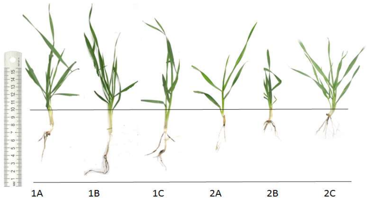
Рис. 2. Диференціація закладання вузла кущіння рослин пшениці різних сортів: 1 – Ювівата 60; 2 – КС 1 (А – Полісся; В – Полісся–Лісостеп; С – Лісостеп)
