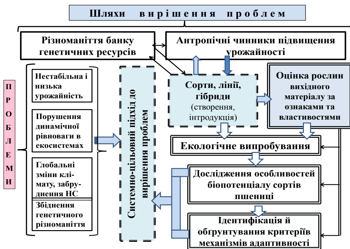
Рис. 1. Алгоритм досліджень
